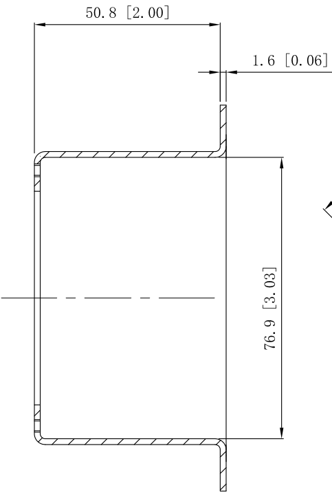
VIEW A-A
