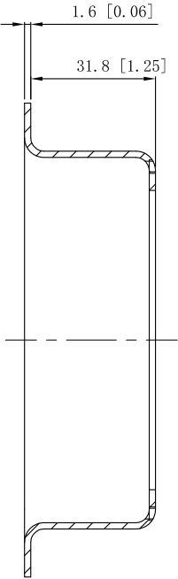
VIEW A-A
