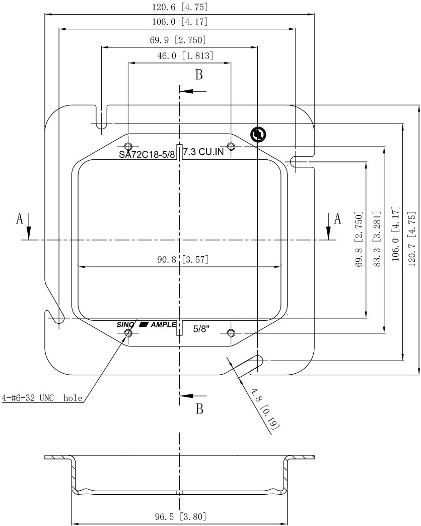
VIEW A-A
