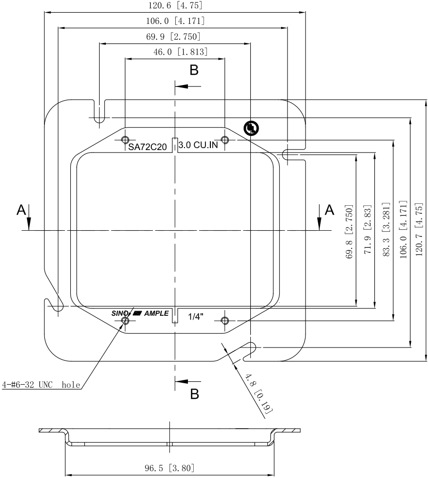
VIEW A-A
