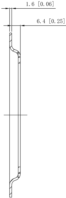
VIEW A-A
